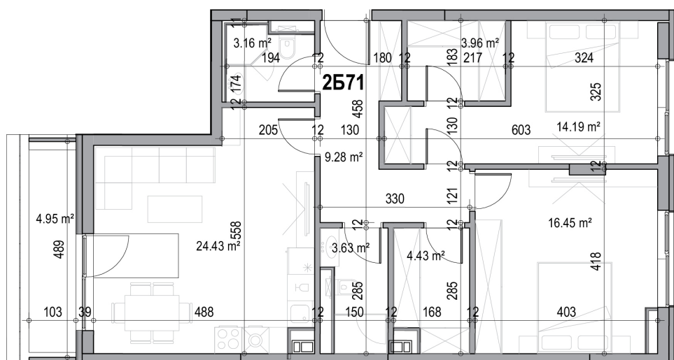
План на апартамента
